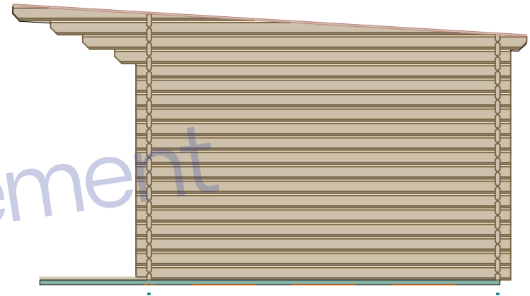
Right Elevation
